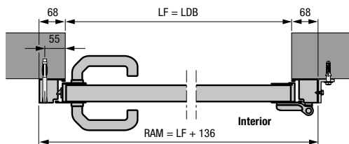
Ușă alăturată cu toc bloc de aluminiu, tip profil 2 Montaj în spatele deschiderii
