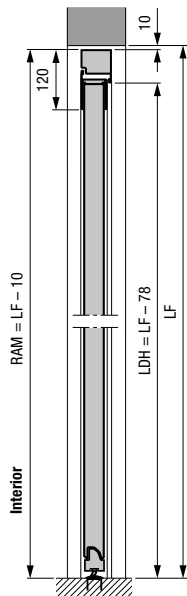
Ușă alăturată cu toc bloc de aluminiu, tip profil 2 Montaj în deschidere
