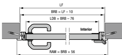
Ușă alăturată cu toc de colț de aluminiu, tip profil 2 Deschidere spre interior
