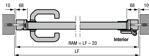
Ușă alăturată cu toc bloc de aluminiu, tip profil 2 Montaj în deschidere
