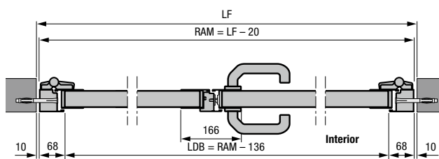
Ușă alăturată cu 2 canaturi și toc bloc de aluminiu, tip profil 2 Montaj în deschidere
