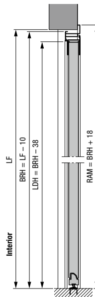
Ușă alăturată cu toc de colț de aluminiu, tip profil 2 Opritor exterior
