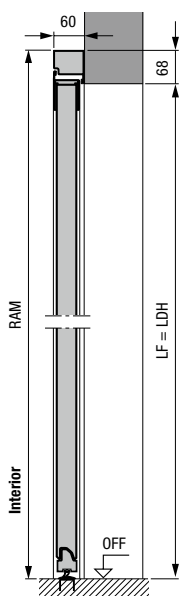
Ușă alăturată cu toc bloc de aluminiu, tip profil 2 Montaj în spatele deschiderii
