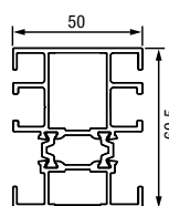
Profil de extensie 50 mm
