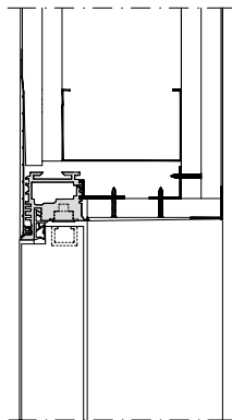
Secțiune verticală cu deschidere inversă în golul ușii (tip RI)
