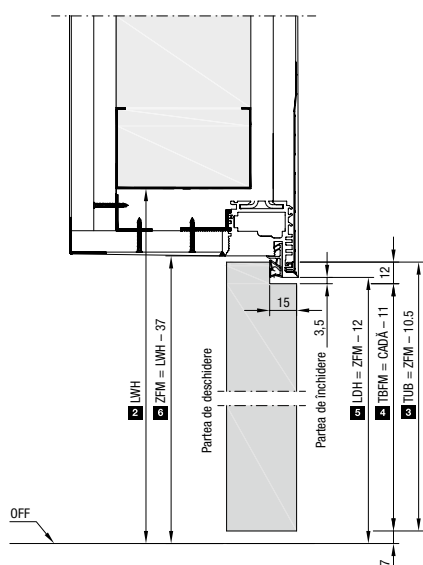
Secțiunea verticală tip RI cu blat ușă cu deschidere inversă
