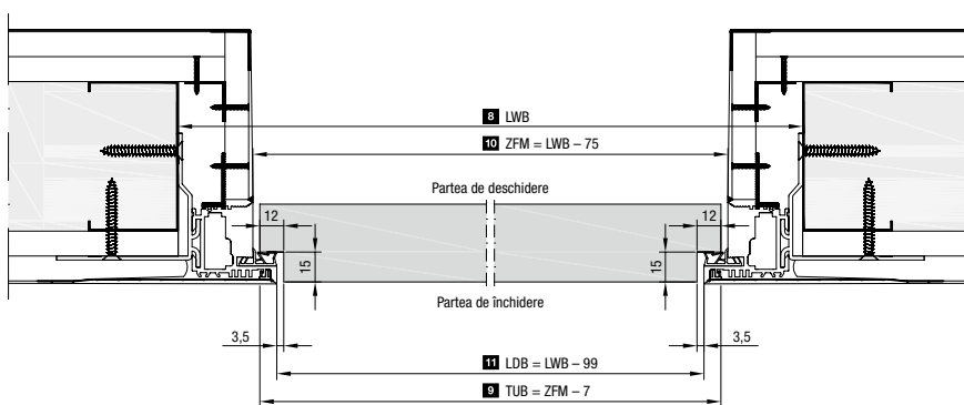
Secțiunea orizontală tip RI cu blat ușă cu deschidere inversă
