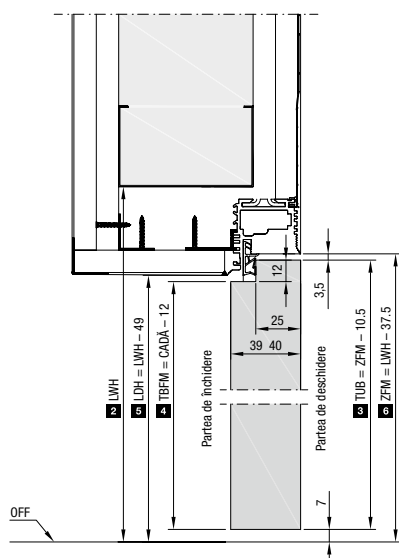
Secțiune verticală tip NA cu blat ușă cu deschidere normală
