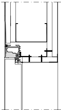
Secțiune verticală cu deschidere normală spre exterior (tip NA)
