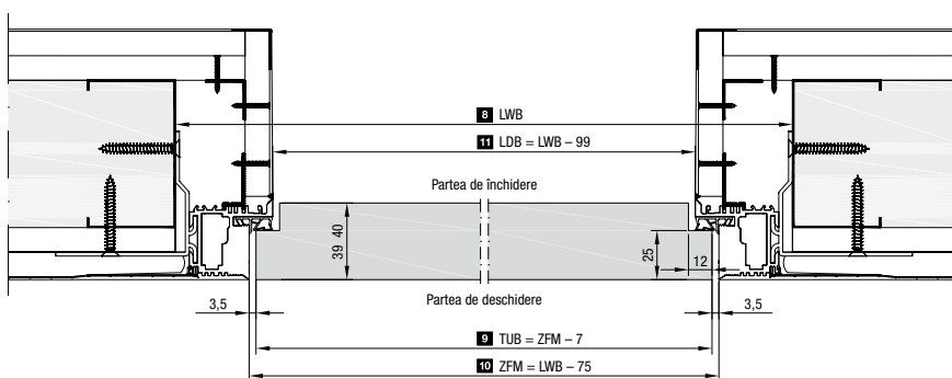
Secțiunea orizontală tip NA cu blat ușă cu deschidere normală
