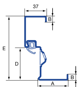
Toc de ușă DryFix
