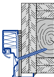
Fixare pe diagonală Perete de compartimentare F90B
