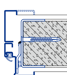
Montare prin sudare BCA (beton celular autoclavizat)
