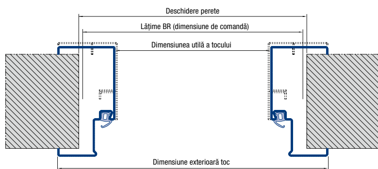
Toc din 3 părți (Uși) Lățime BR Înălțime BR
