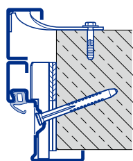
Fixare pe diagonală Zidărie
