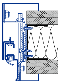
Montaj mascat Perete de compartimentare F90A
