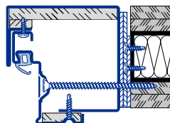
Montaj cu șuruburi Perete de compartimentare F90A
