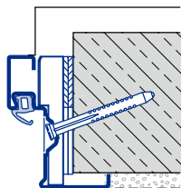
Fixare pe diagonală Zidărie
