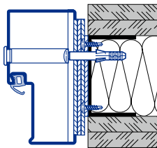
Montaj cu șuruburi Perete de montaj F90A
