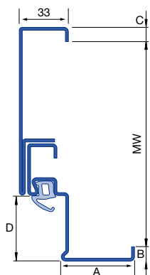
Toc de îmbrăcare a zidului cu 2 cochilii
