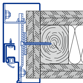
Montaj mascat Perete de compartimentare F 90 B
