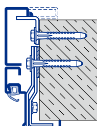
Montaj intrados Zidărie
