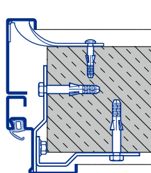
Montaj peste colțul peretelui Zidărie
