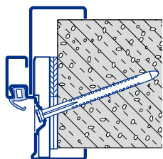
Fixare pe diagonală Zidărie / beton / BCA (beton celular autoclavizat)
