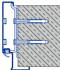
Montaj mascat Beton aparent / zidărie aparentă
