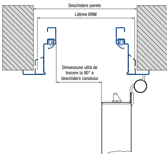
Ușă cu 1 canat
