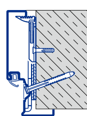
NOU. Fixare pe diagonală Beton aparent / zidărie apărentă până la MW 450
