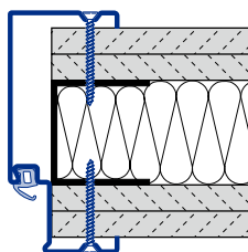
Montaj cu șuruburi Perete de compartimentare F90A
