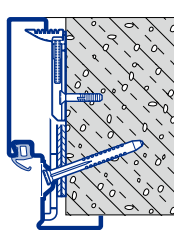
NOU. Fixare pe diagonală BCA (beton celular autoclavizat) până la MW 450
