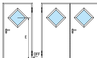
Vitrare în romb
