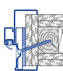
Fixare pe diagonală Perete de compartimentare F 90 B
