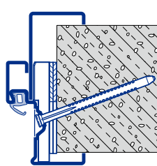
Fixare pe diagonală BCA (beton celular autoclavizat)
