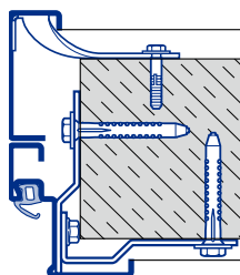
Montaj intrados Zidărie
