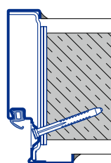
Fixare pe diagonală Beton aparent / zidărie apărentă până la MW 175
