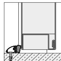
Șină de oprire din aluminiu cu etanșare și profil de protecție, tip C2
