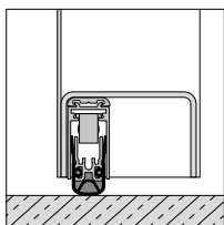
Garnitură retractabilă de etanșare la pardoseală, hidrolică, timp întârziat, tip A2
