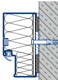
Montaj cu dibluri Zidărie tencuită
