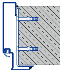
Montare prin sudare Beton aparent / zidărie aparentă
