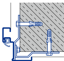
Montaj peste colțul peretelui Zidărie
