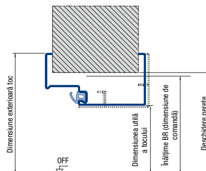
Toc din 4 părți (Ușă) Lățime BR Înălțime BR
