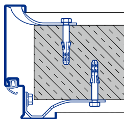
Montaj cu dibluri Zidărie tencuită
