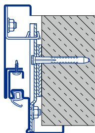
Montaj mascat Beton aparent / zidărie aparentă
