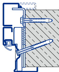
Fixare pe diagonală Zidărie aparentă / beton aparent
