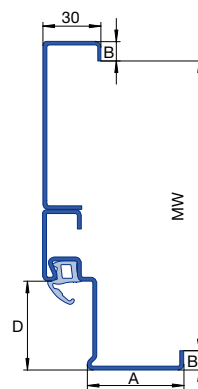
Toc de colț cu toc complementar
