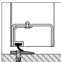
Profil inferior de închidere din aluminiu cu etanșare și prag curbat tip B1
