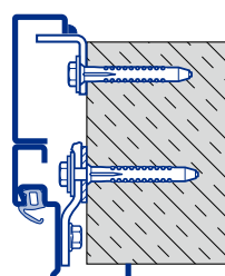
Montaj mascat Zidărie
