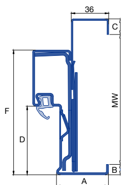
Toc DryFix cu toc complementar Vario B36 până la RC 2
