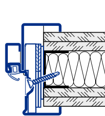
Fixare pe diagonală Perete de compartimentare F90A
