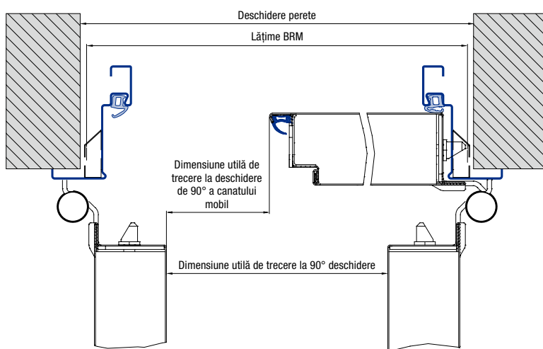
Ușă cu 2 canaturi
