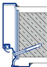
Fixare pe diagonală BCA (beton celular autoclavizat) până la MW 175
