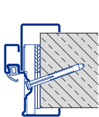
Fixare pe diagonală Zidărie / beton aparent
