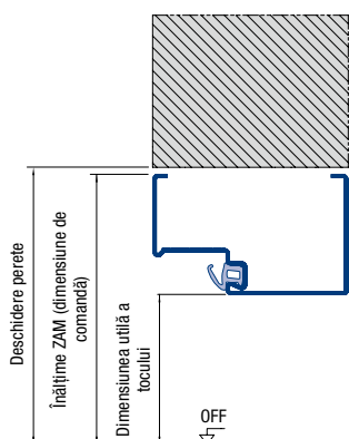
Toc din 4 părți (Ușă) Lățime ZAM Înălțime ZAM
