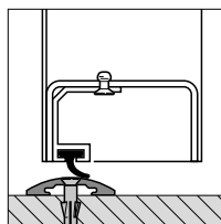
Profil inferior de închidere din aluminiu cu etanșare și prag semirotund tip B2
