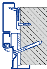
Fixare pe diagonală Zidărie aparentă / beton aparent
