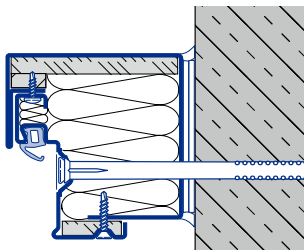
Montaj cu dibluri Zidărie
