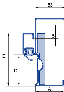
Toc de colț cu toc complementar Vario B53
