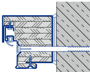
Montaj cu dibluri Zidărie
