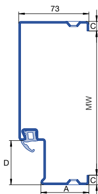
Toc de îmbrăcare a zidului B73 pentru perete despărțitor
