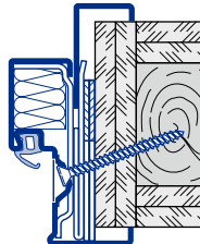
Fixare pe diagonală Perete de montaj F90B
